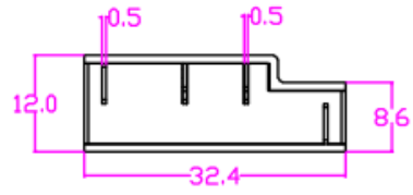
底视图
