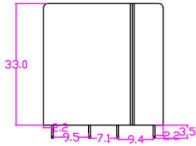
正面图
