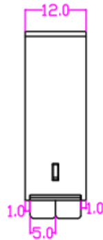
L/N/PE铜脚侧面图
